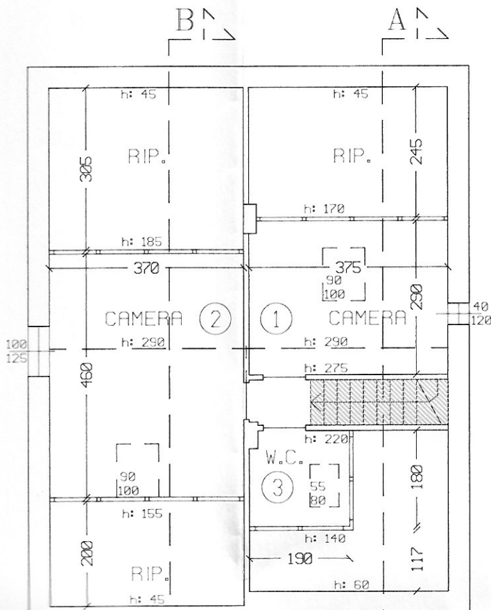
PIANTA SOTTOTETTO - stato in progetto
