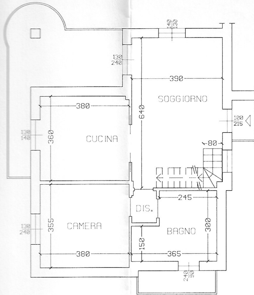
PIANTA PIANO PRIMO - stato in progetto
